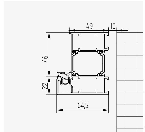
WYMIAROWANIE OŚCIEŻNICY
