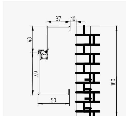
WYMIAROWANIE OŚCIEŻNICY
