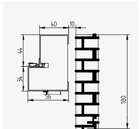
WYMIAROWANIE OŚCIEŻNICY
