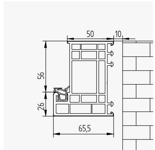
WYMIAROWANIE OŚCIEŻNICY
