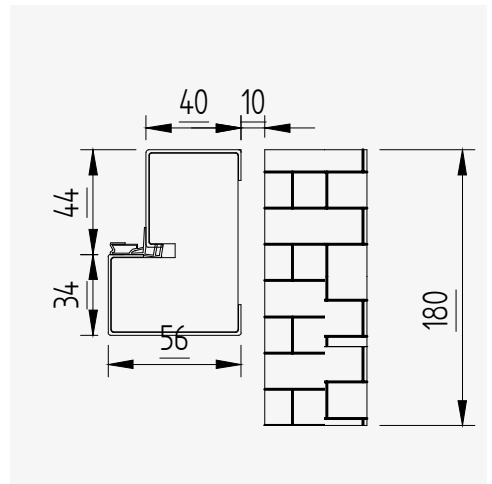
WYMIAROWANIE OŚCIEŻNICY
