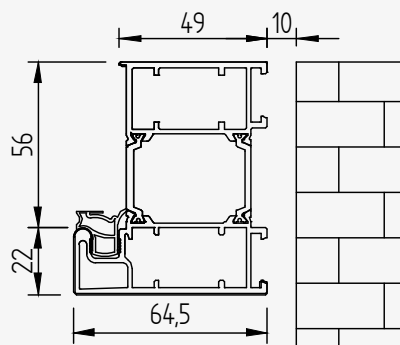
WYMIAROWANIE OŚCIEŻNICY
