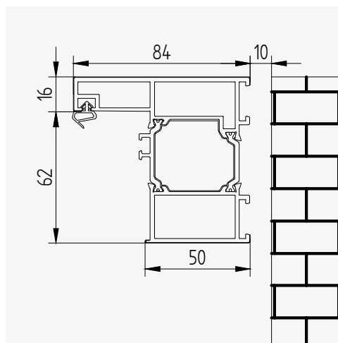
WYMIAROWANIE OŚCIEŻNICY
