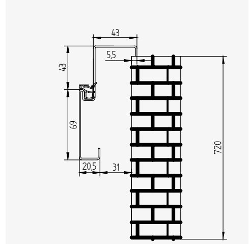
WYMIAROWANIE OŚCIEŻNICY
