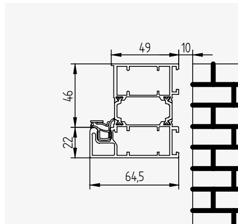
WYMIAROWANIE OŚCIEŻNICY
