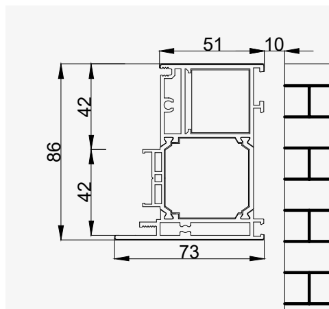
WYMIAROWANIE OŚCIEŻNICY
